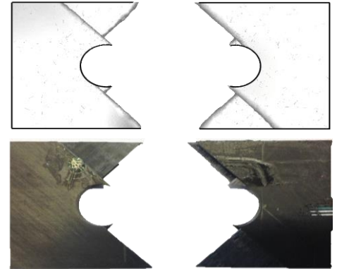
Figure: Rupture d'un laminé [45/-45]S prédite par une combinaison MFH pour la rupture intralaminare et éléments cohésifs pour la rupture inter-laminare (haut) et observée expérimentalement (bas) [WU15]
